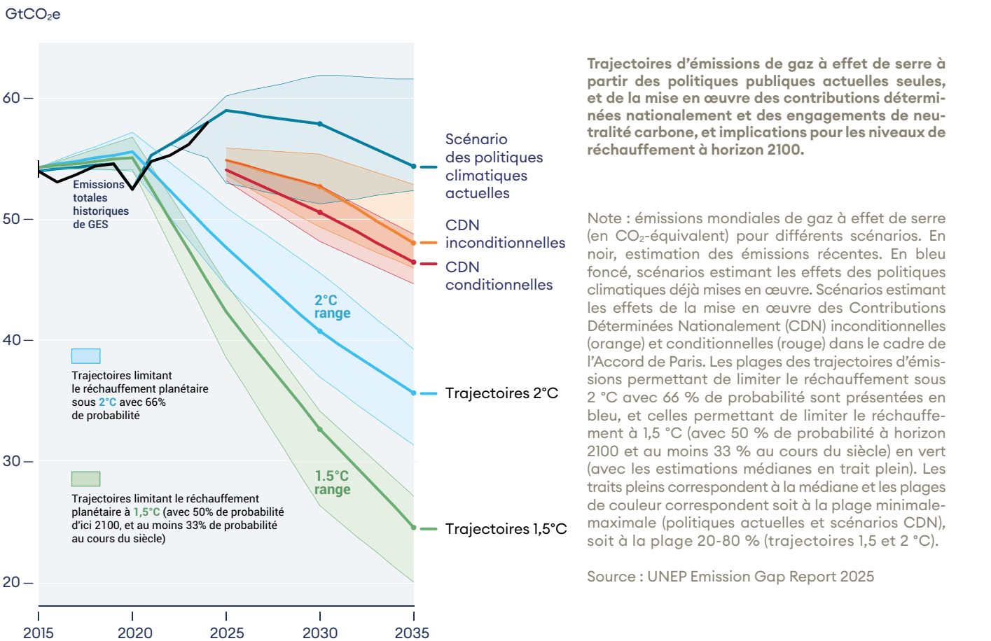
Figure 2.3.2.a – Trajectoires d'émissions de gaz à effet de serre selon différents scénarios et implications pour les niveaux de réchauffement planétaires à horizon 2100
